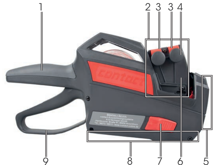
Abbildung 1 Handauszeichner geschlossen - Seitenansicht
